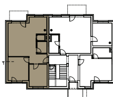
PÔDORYS PODLAŽIA
