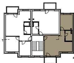
PÔDORYS PODLAŽIA
